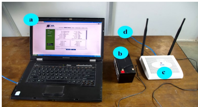
Fig 1 Measurement setup (a) Laptop (b) +12V battery (c) CPE (d) RJ-45 Ethernet cable
