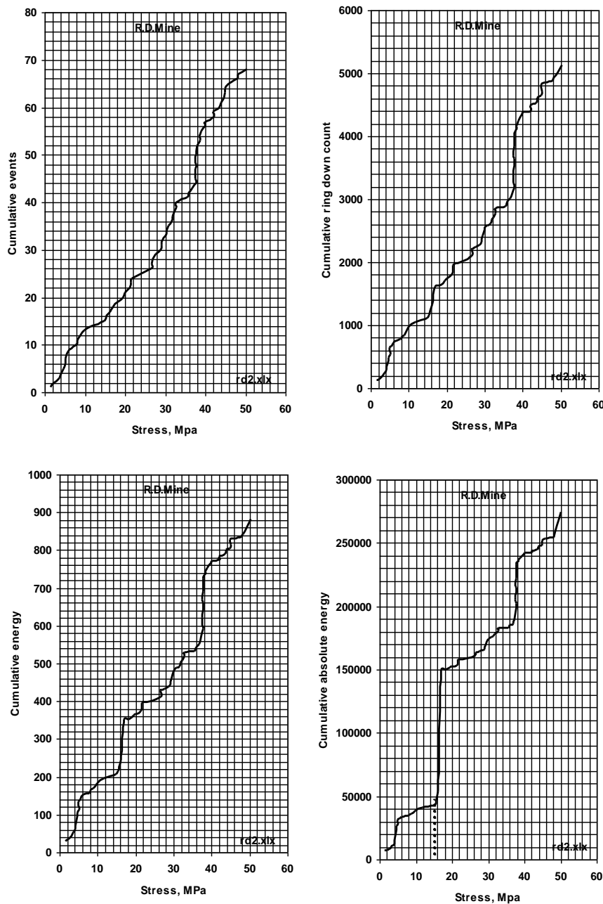
Figure 5. AE parameter plots for site-2
