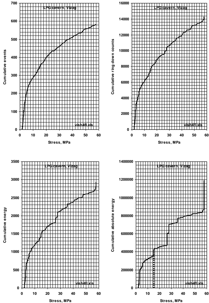
Figure 6. AE parameter plots for site-3
